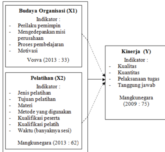
Gambar 1. Kerangka Konsep
